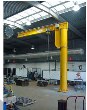
Potences sur fût
